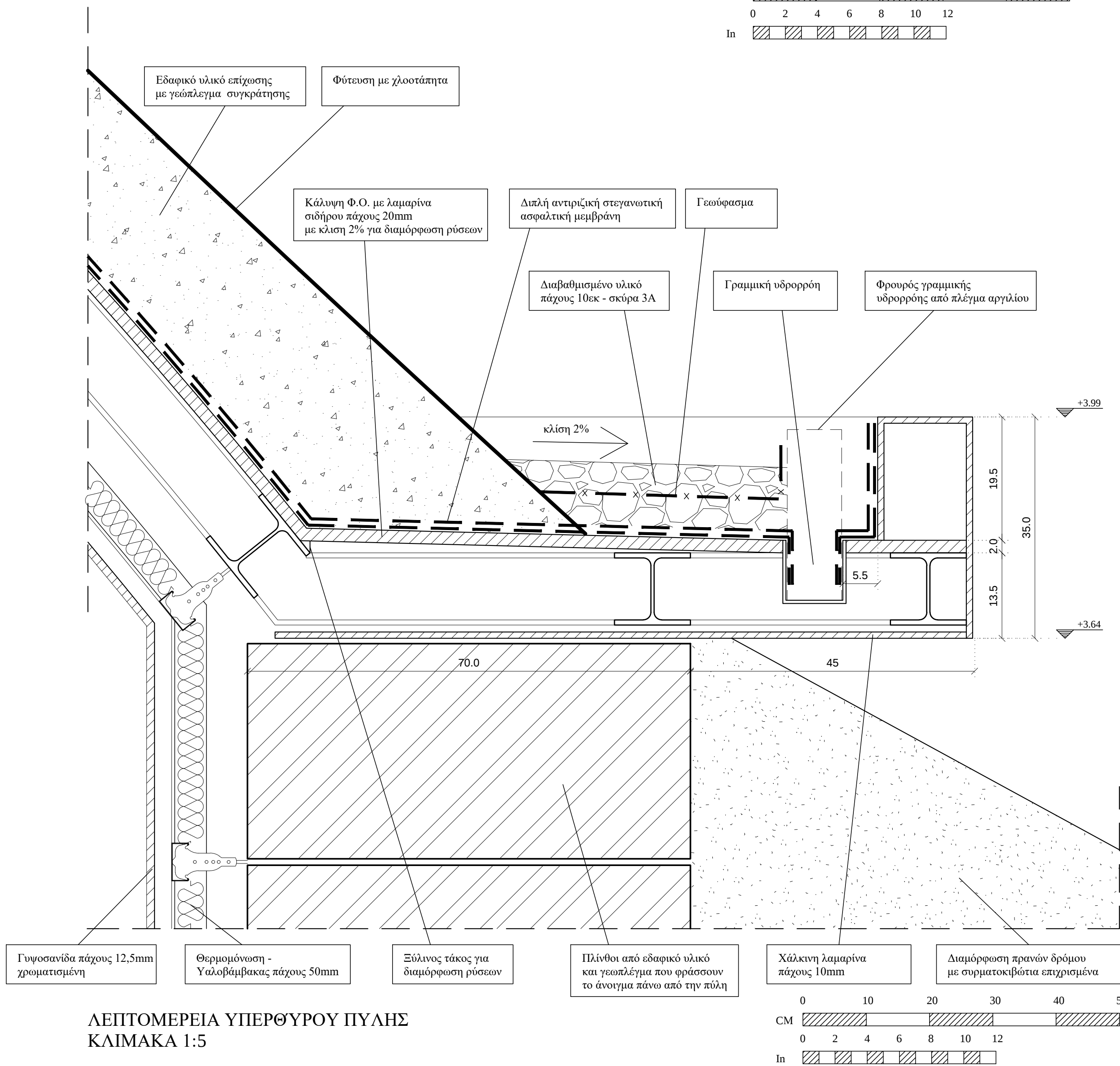
ΛΕΠΤΟΜΕΡΕΙΑ ΥΠΕΡΘΥΡΟΥ ΕΙΣΟΔΟΥ ΣΤΕΓΑΣΤΡΟΥ ΚΛΙΜΑΚΑ 1:5
